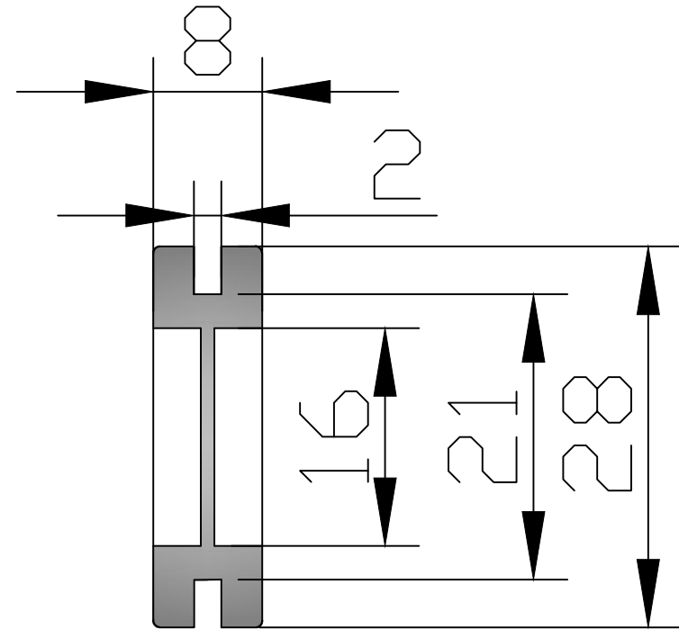
Sezione A-A
